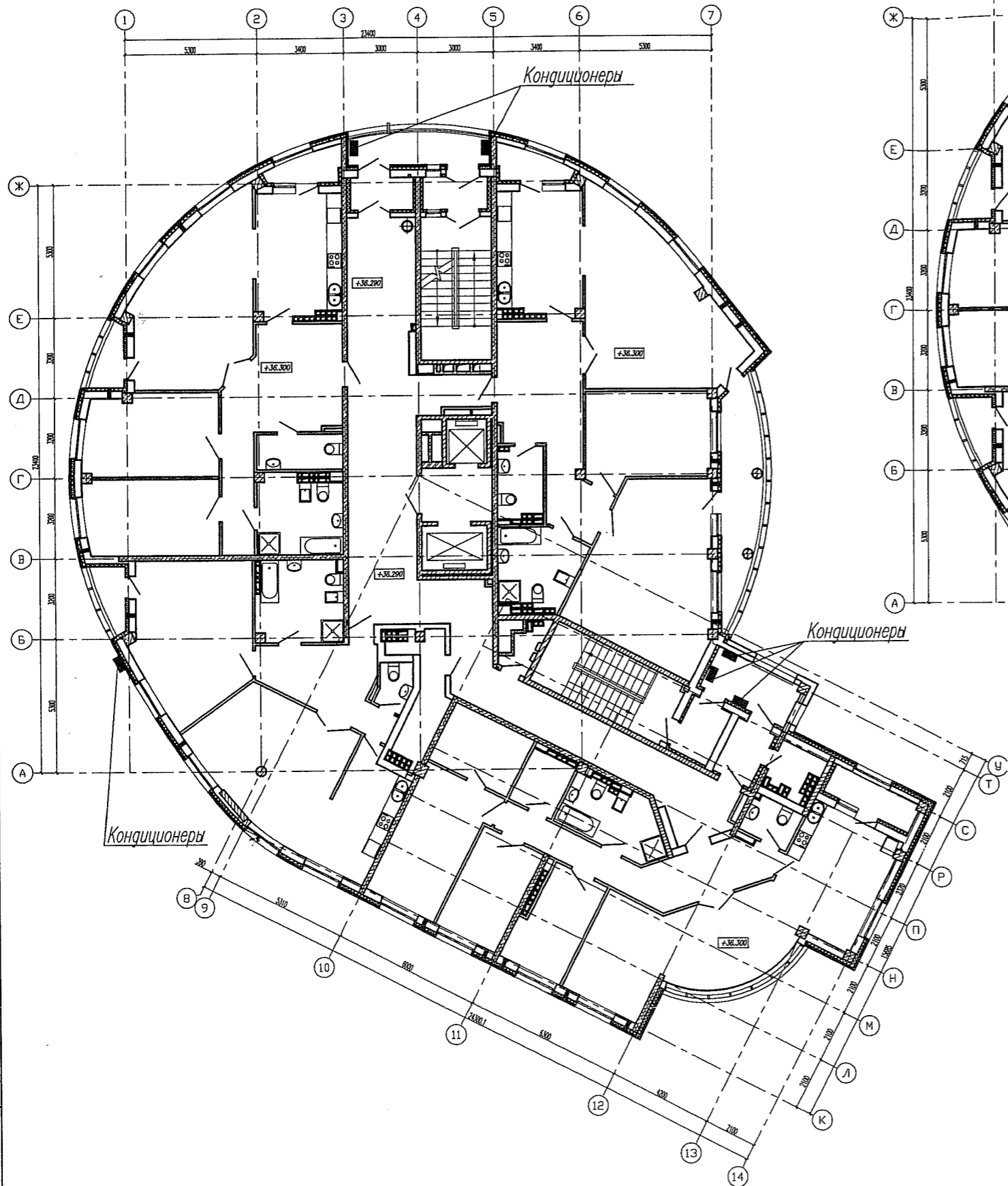
План 12 этажа
