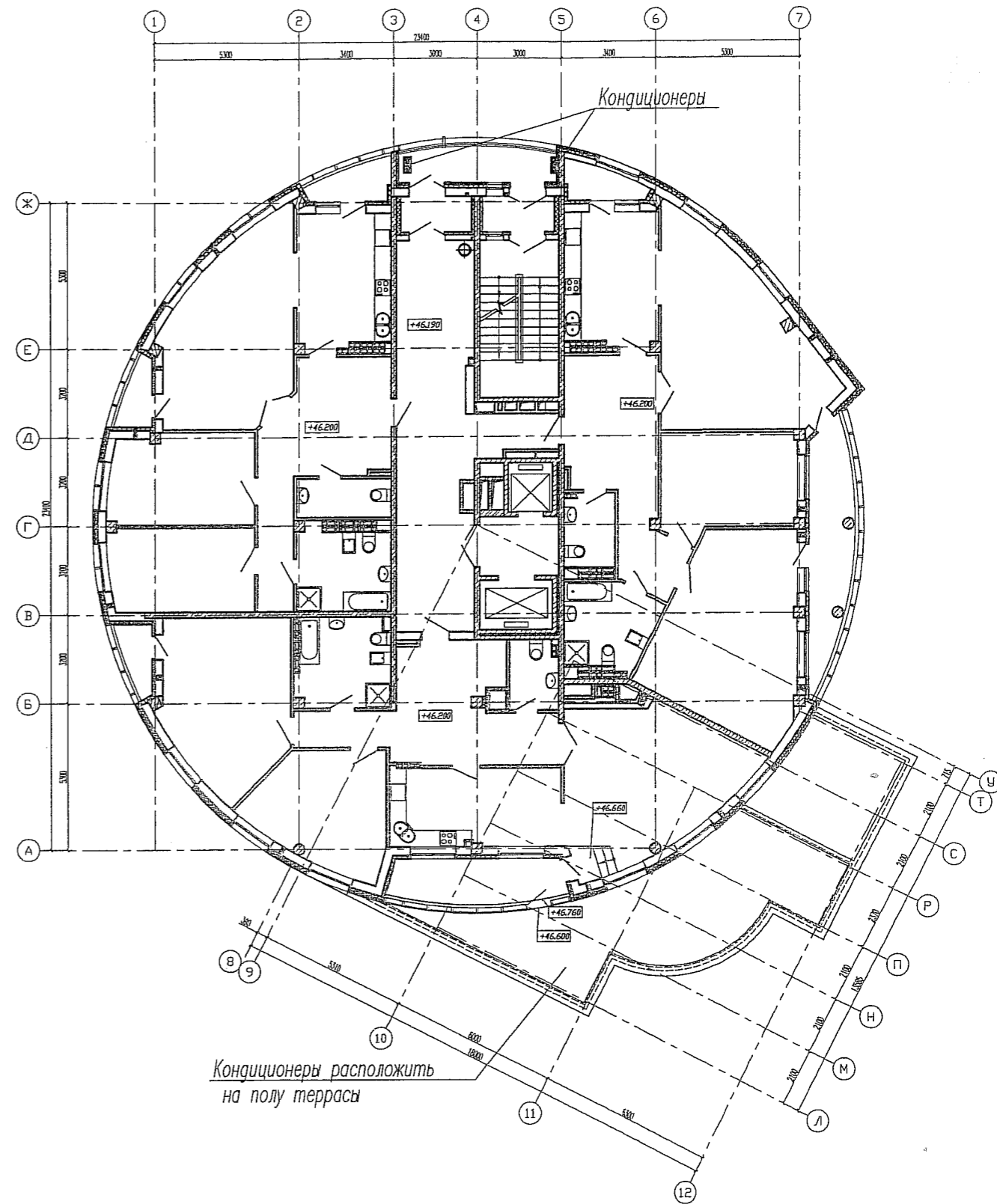
План 15 этажа
