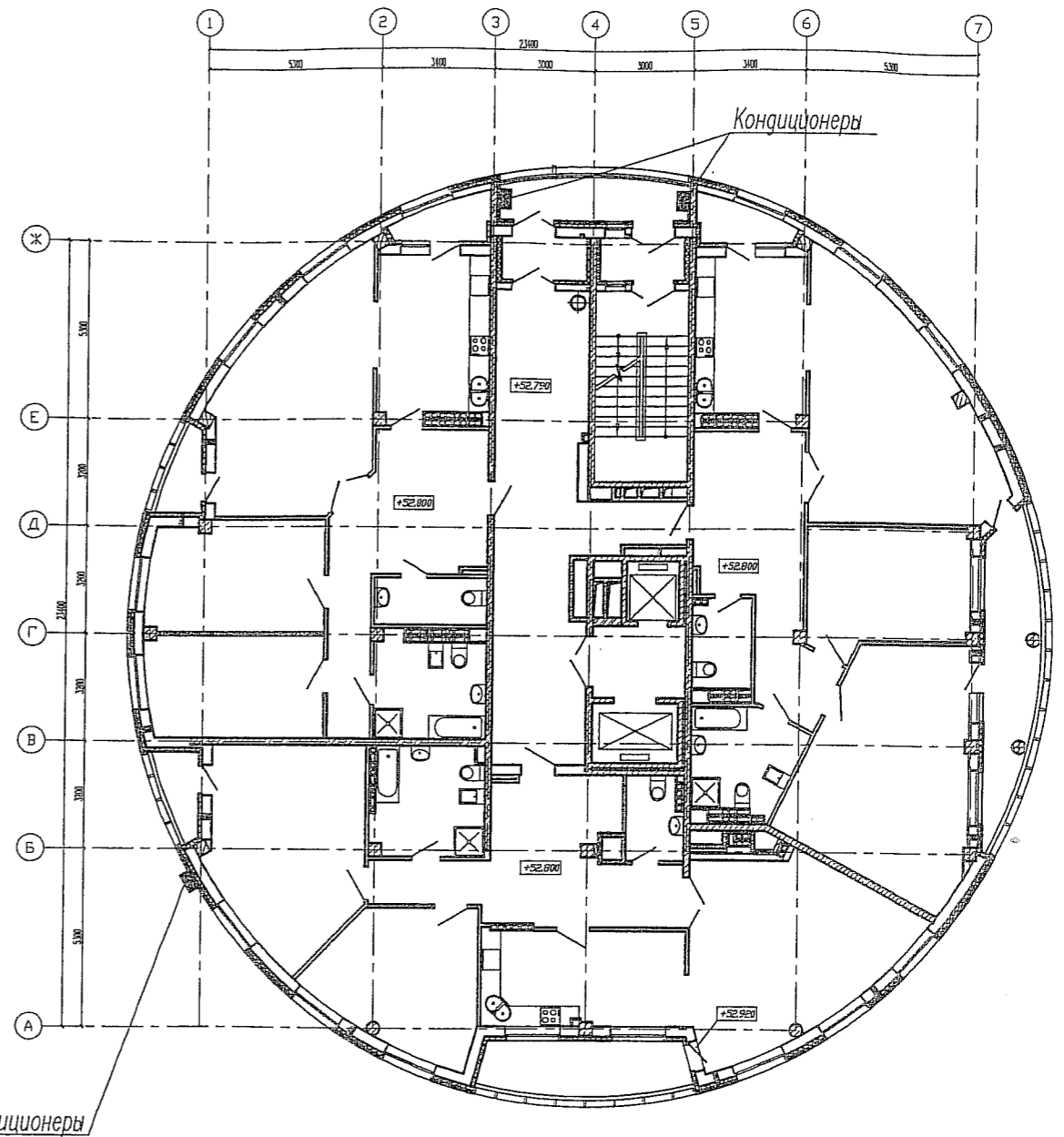
План 17 этажа
