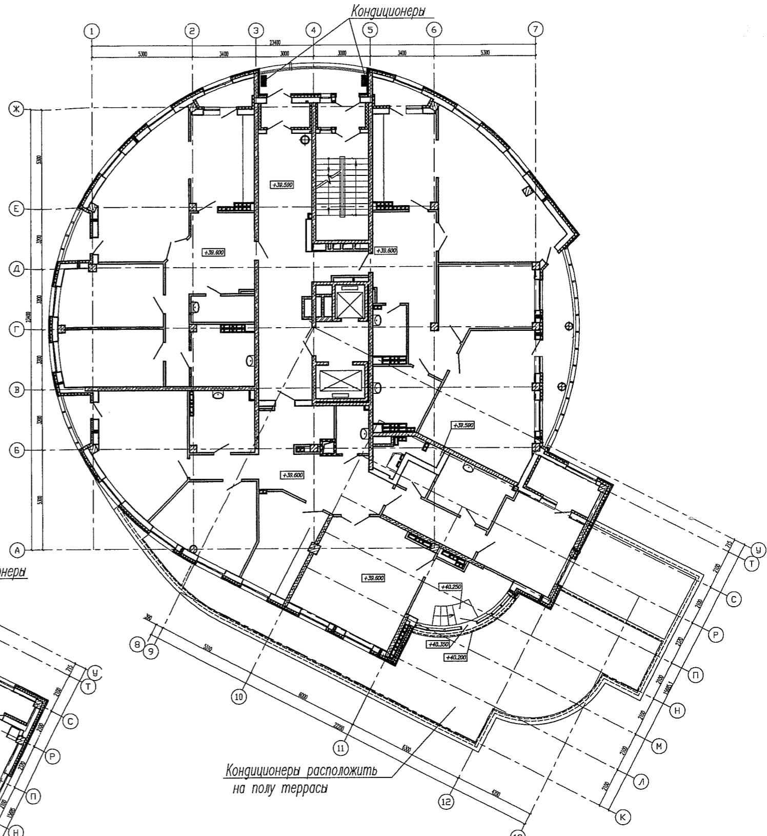
План 13 этажа
