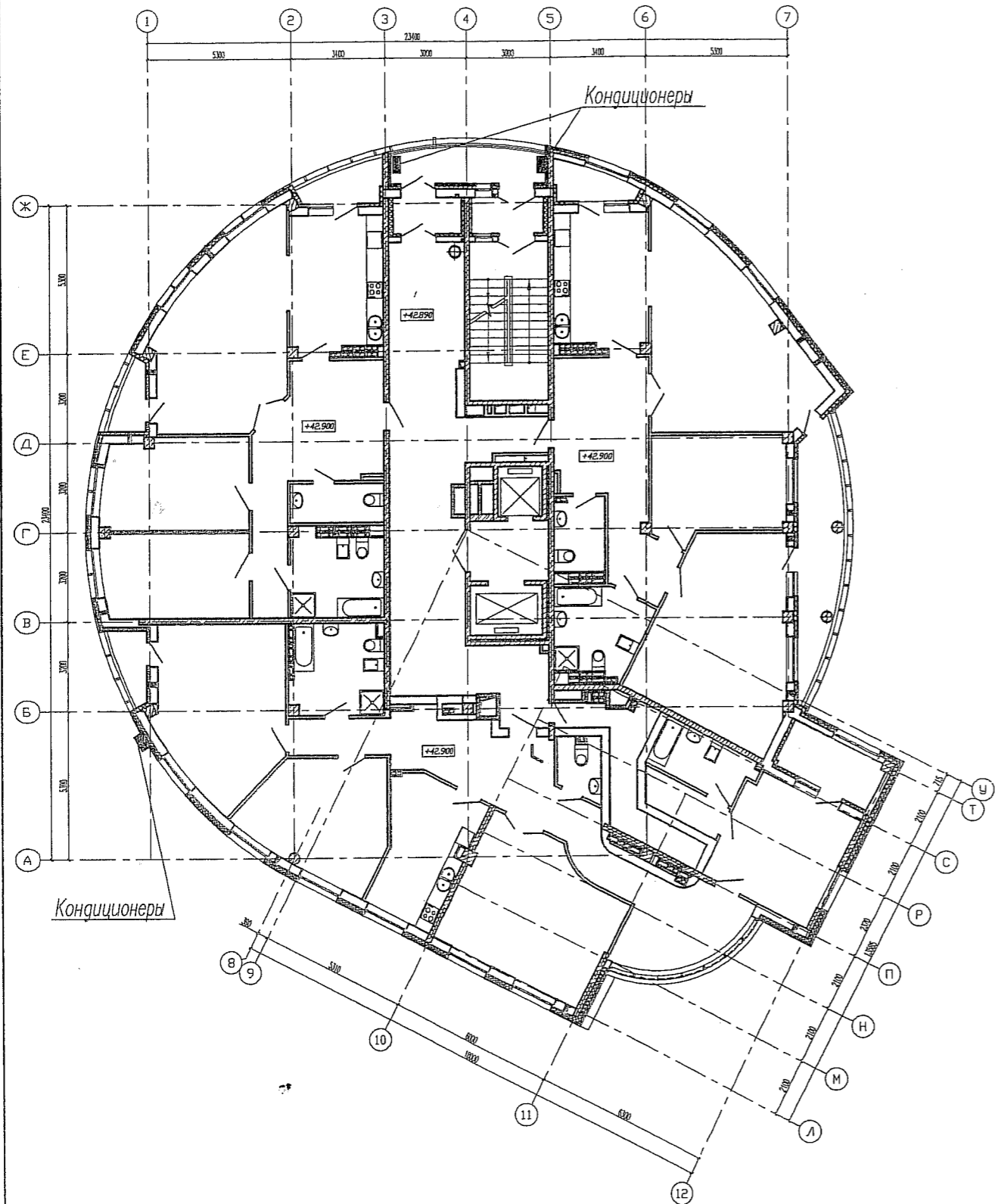
План 14 этажа
