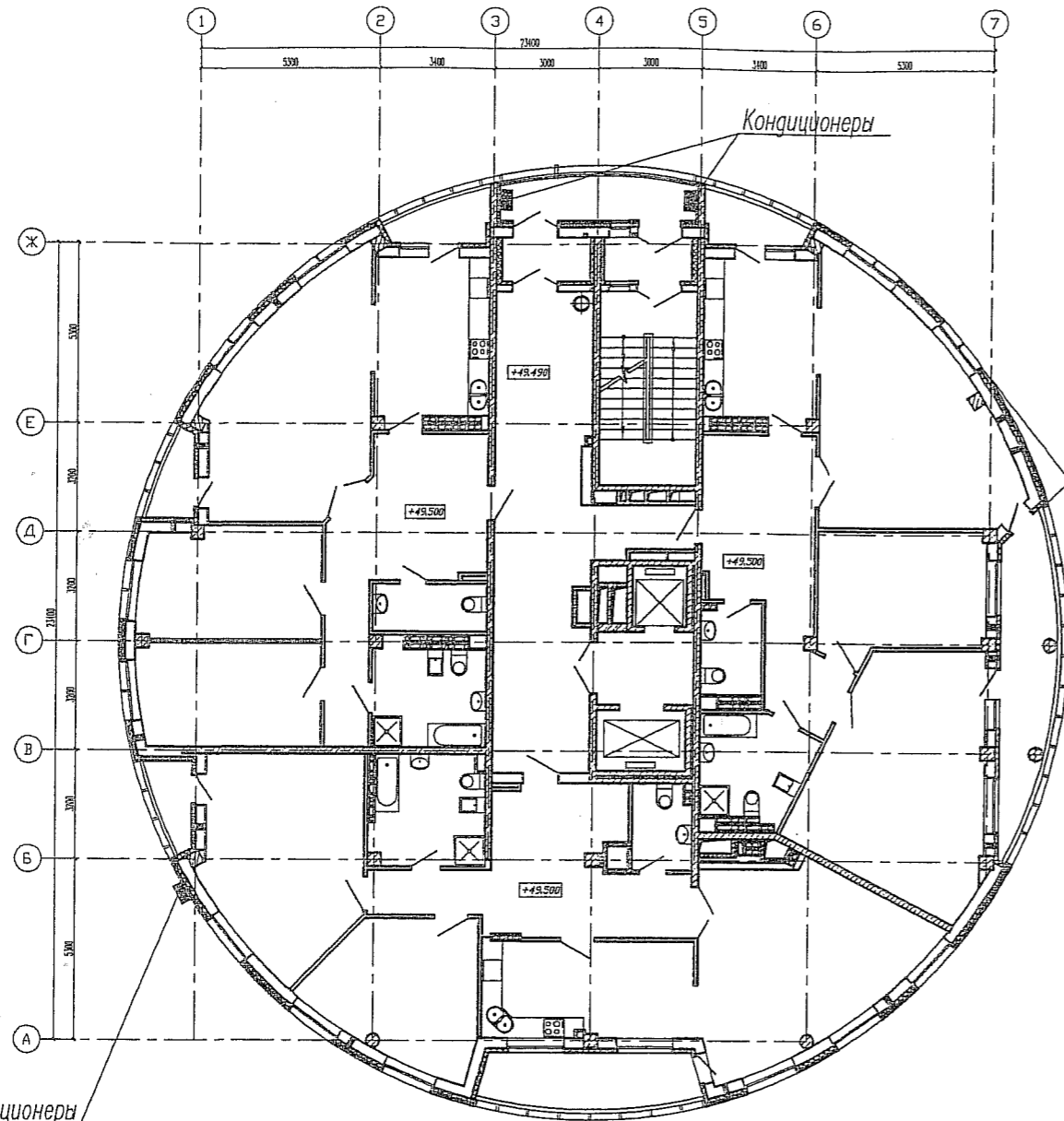
План 16 этажа
